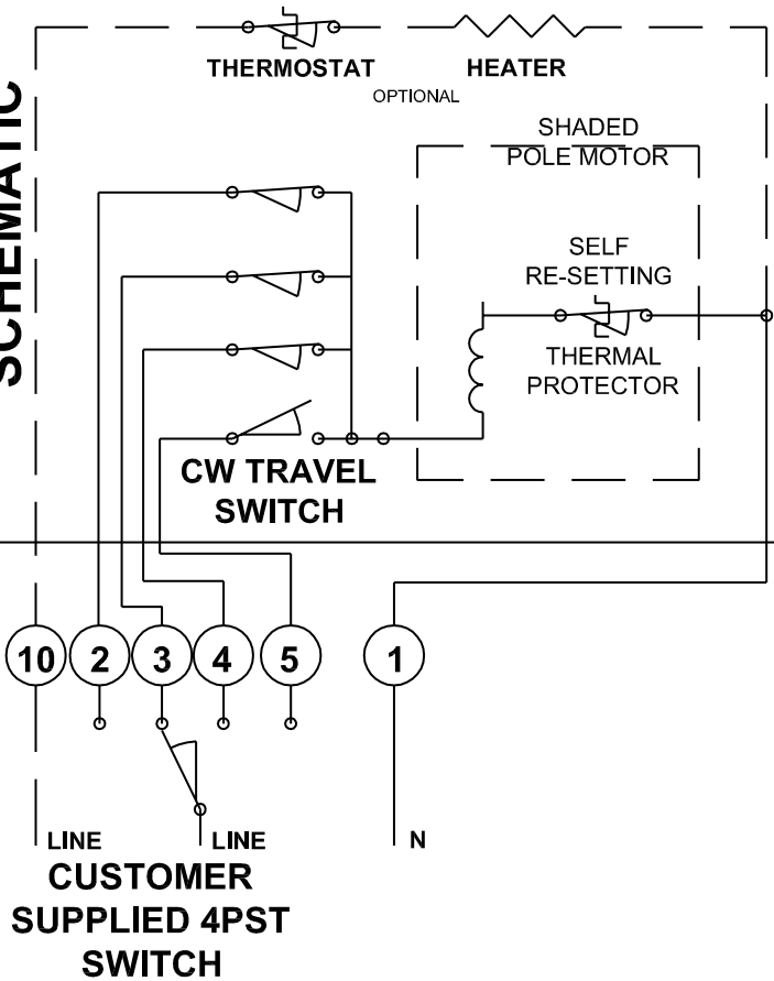
WIRING SCHEMATIC
