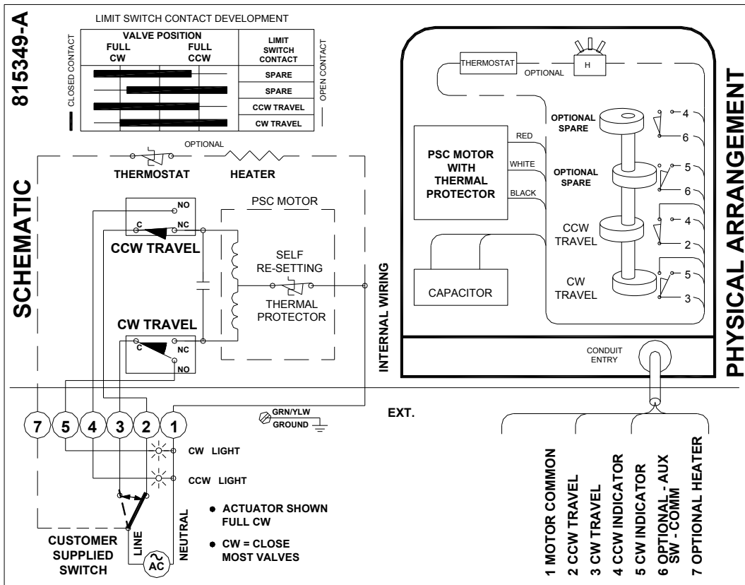
WIRING SCHEMATIC
